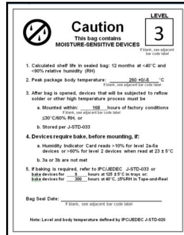
MSL3 Label
